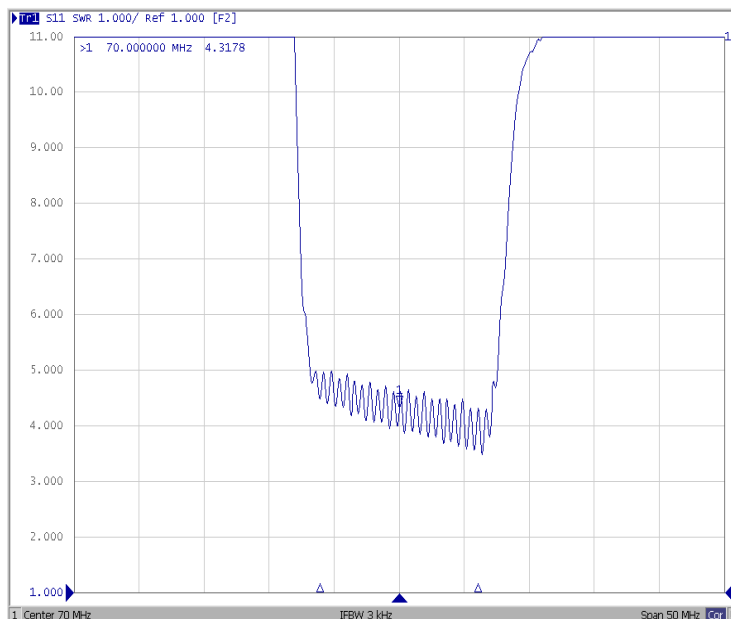
VSWR S11
